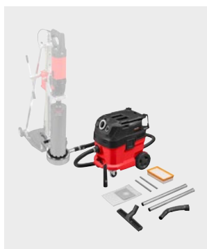
Sugning af boreslam ved vådboring med ROLLER'S borestandere
