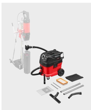
Saugen von gesundheitsgefährdenden Stäuben beim Trockenbohren
