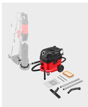
Saugen von Bohrschlamm beim Nassbohren mit ROLLER'S Bohrstäben
