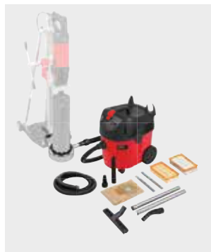
Saugen von Bohrschlamm beim Nassbohren mit ROLLER'S Bohrständern
